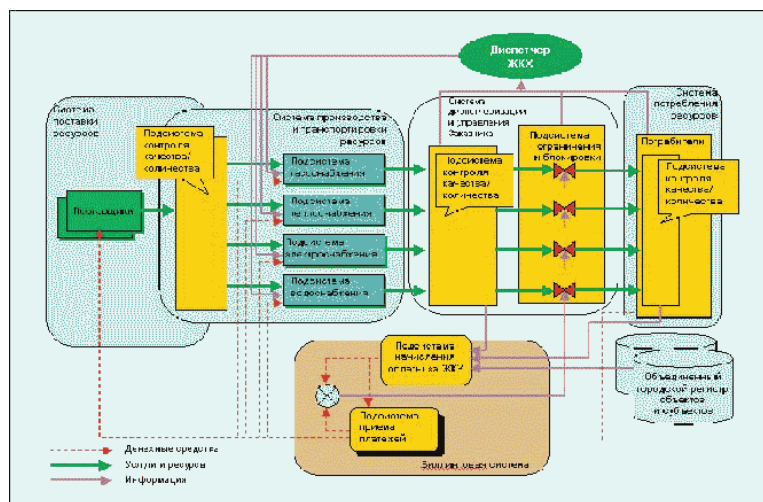
Рис. 17. Диспетчеризация на уровне учреждения эксплуатации городского хозяйства
